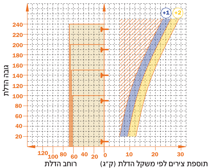
חישוב מספר הצירים שיש להרכיב בהתאם למידות ומשקל הדלת
