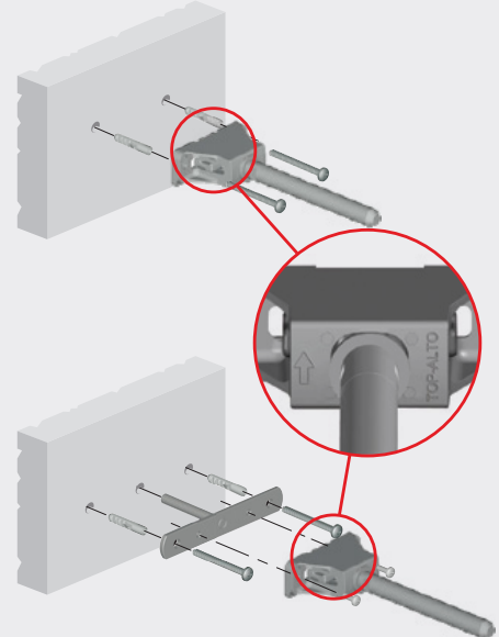
TRIAD MAXI – התקנה עם בסיס חיזוק
