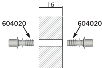
התקנת הבורג בדופן משותפת
