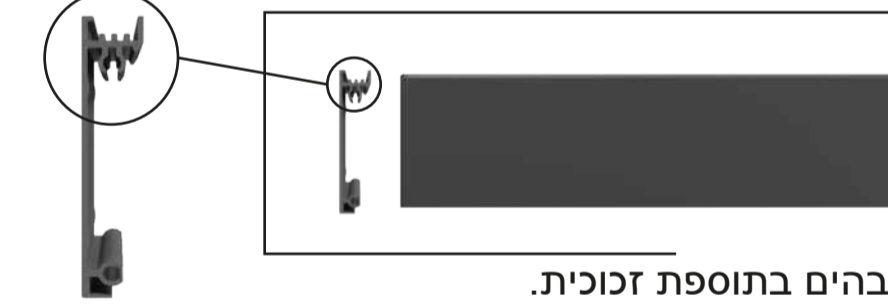
פרופיל אלומיניום גובה 62 מ"מ המתאים לחזית אלומיניום עבור שלושת הגבהים בתוספת זכוכית.
