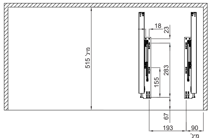
מידות התקנה מימין
