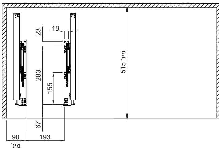
מידות התקנה משמאל
